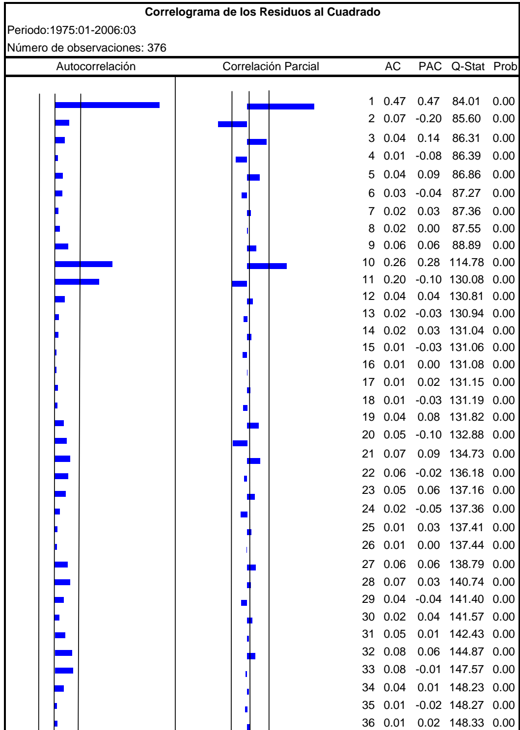
Gráfico 2: Correlograma de los residuos al cuadrado
